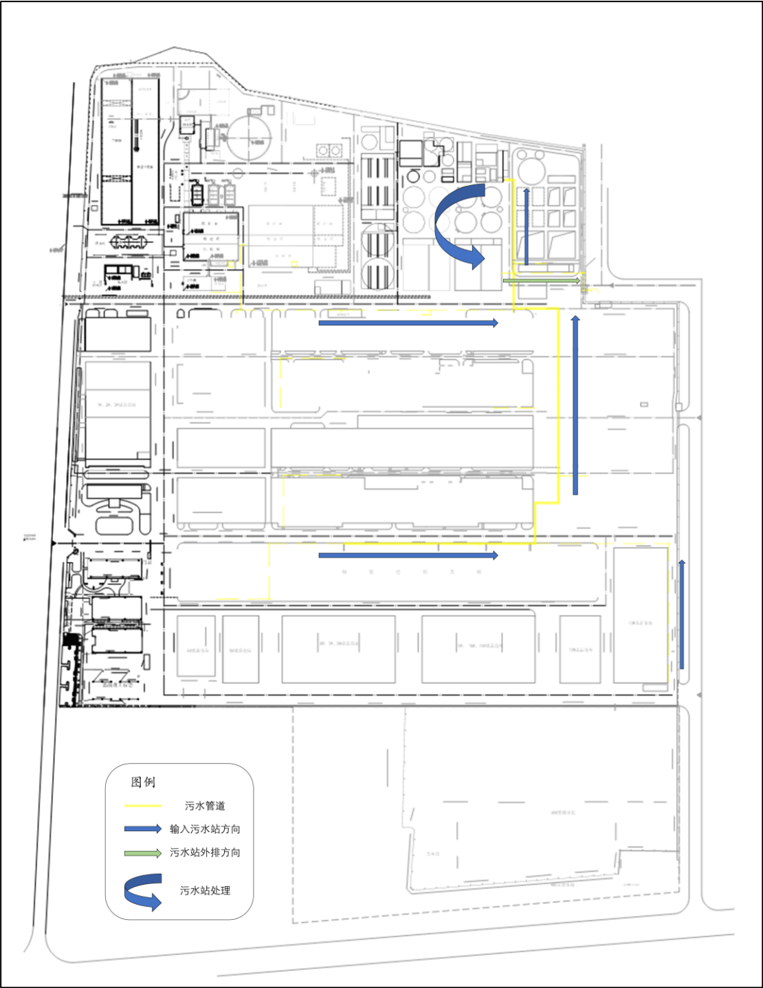
图 11-7 污水管网图
