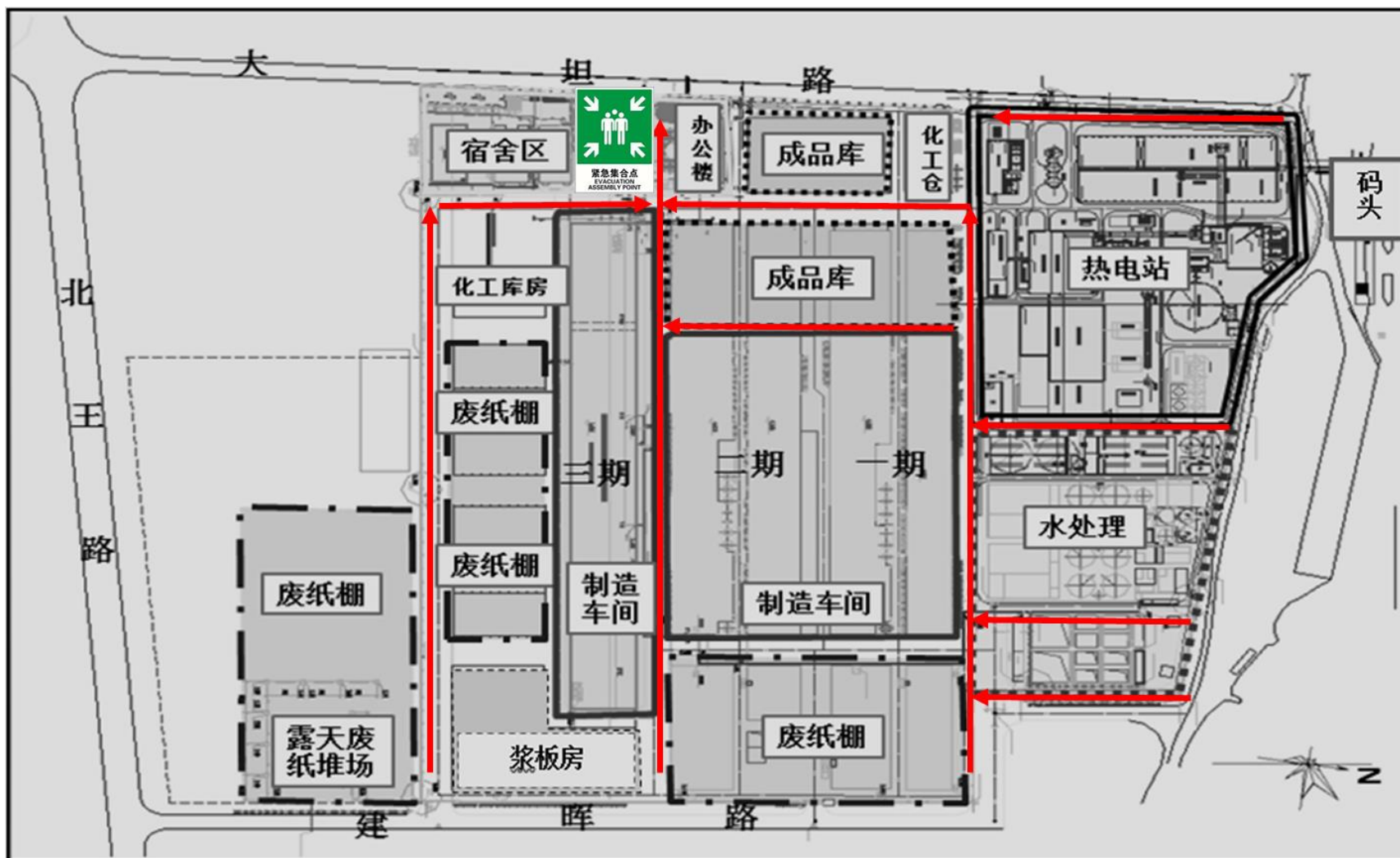
图 11-5 疏散示意图
